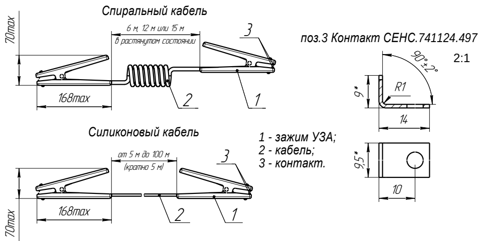
Рисунок 6 – Заземляющий проводник
