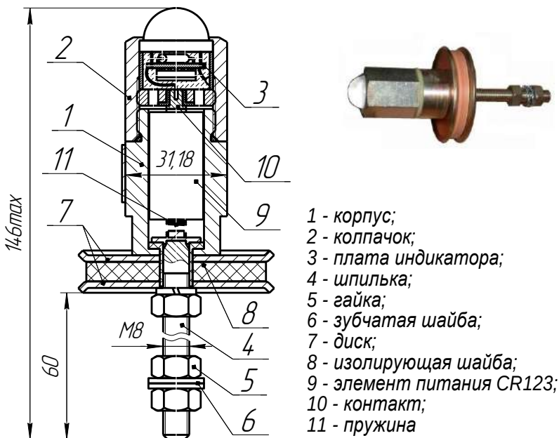
Рисунок 5 – Индикатор
