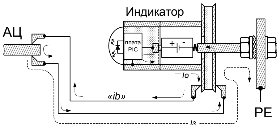
Рисунок 3 – Схема соединений
