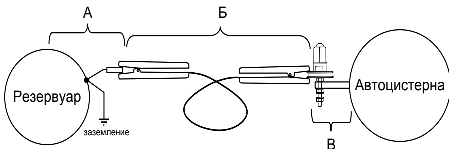
Рисунок 10 – Цепь заземления при установке индикатора на автоцистерне (по рисунку 2)
