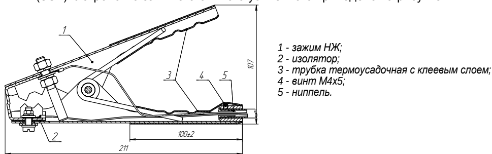
Рисунок 7 – ЗСТ – зажим стальной усиленный
